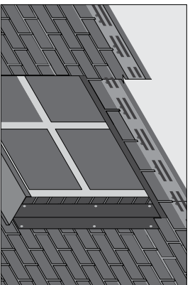
Рис. 8.4. Монтаж оконного наличника сверху проема
