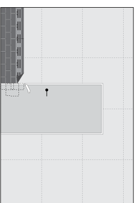
Рис. 7.1. Монтаж фасадной плитки вокруг дверных проемов
