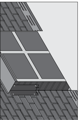
Рис. 8.3. Монтаж оконного наличника сбоку проема
