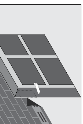
Рис. 8.1. Монтаж фасадной плитки вокруг оконных проемов
