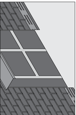
Рис. 8.2. Установка подоконного отлива
