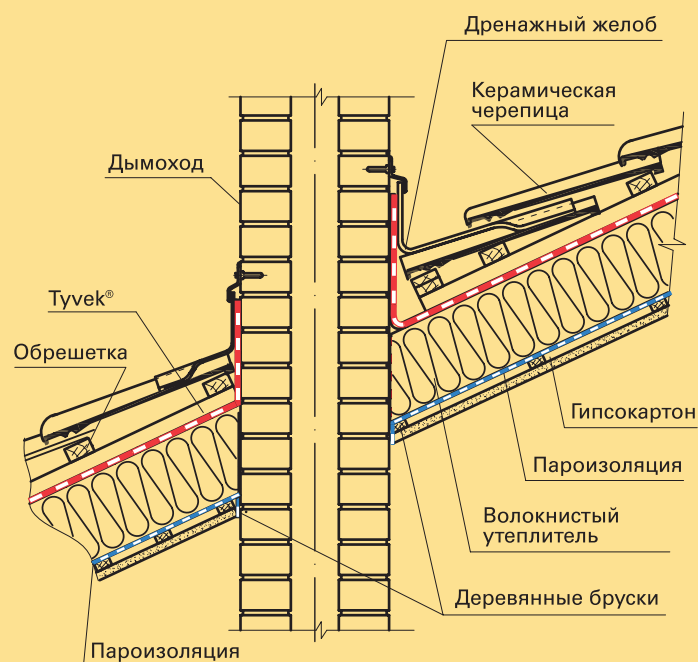
Рис. 3 Дымоход
