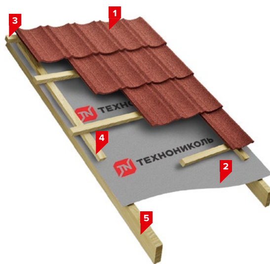
Рис. 5. Строение кровельной системы ТН-ЛЮКСАРД Классик
